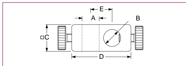
07 CFL 直角ポストクランプ
