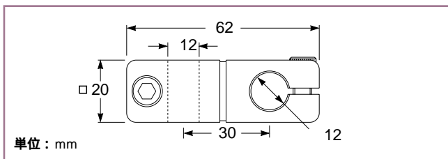
07 CFH ヘビーデューティ直角ポストクランプ
