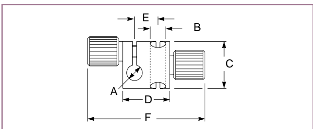
07 CFG 直角ポストクランプ
