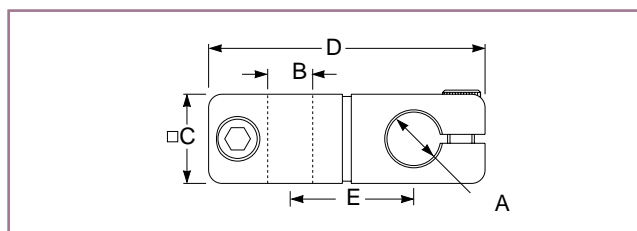
07 CFH ヘビーデューティ直角ポストクランプ
