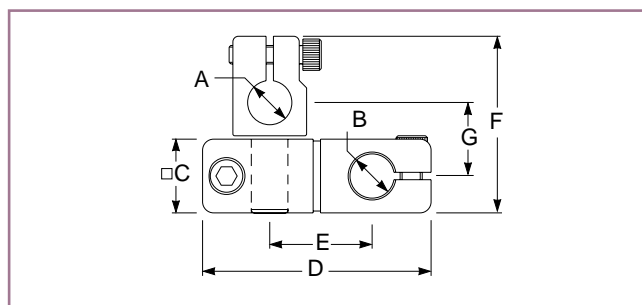
07 CRH ヘビーデューティアジャスタブル ポストクランプ
