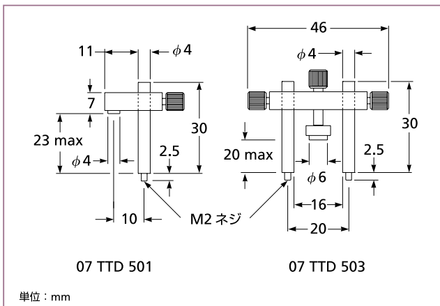
07 TTD 501および503 光学部品用リテーナ
