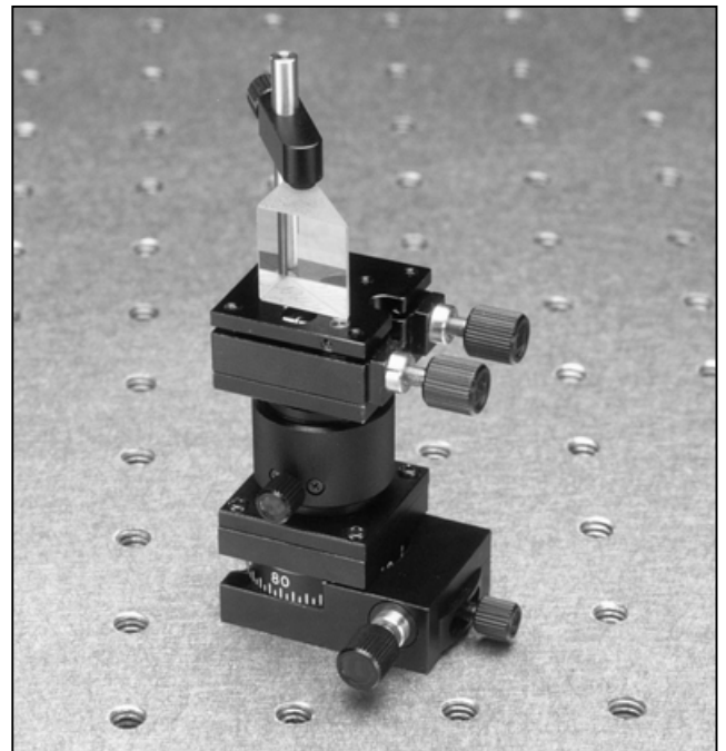
薄型傾斜ステージに取付けられたプリズム
