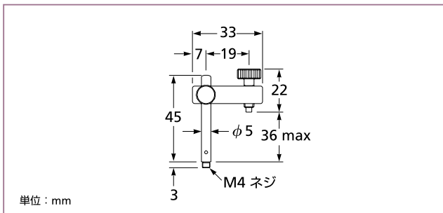
07 TTD 001 光学部品用リテーナ
