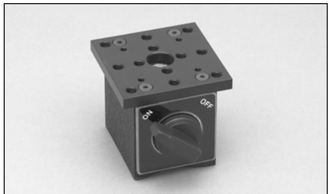
07 BMS 001 マグネチックベースに取り付けられた 07 BMA 501 トッププレート
