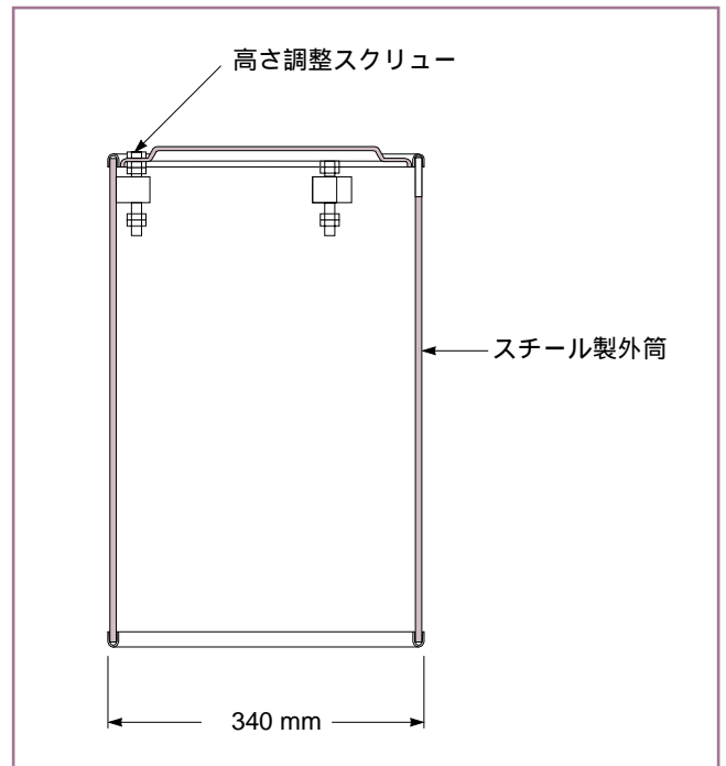
除振機能の無い固定サポート
