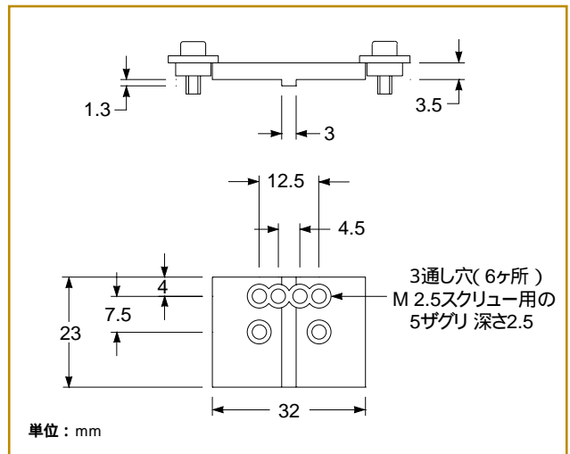
17 ASA 001 アダプタープレート
