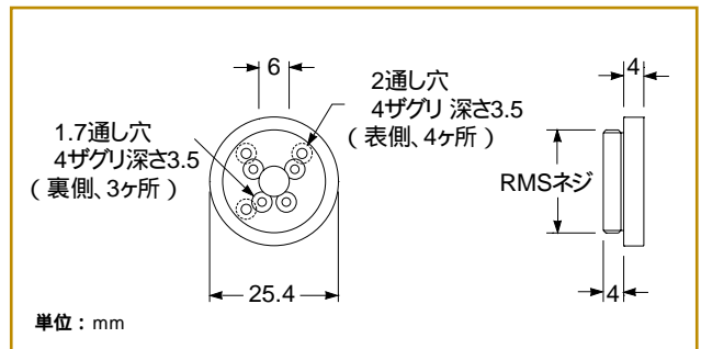
17 ASA 003 アダプタープレート
